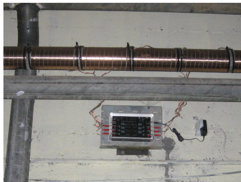
Vulcan S100 安装在一个水表和电表生产厂
