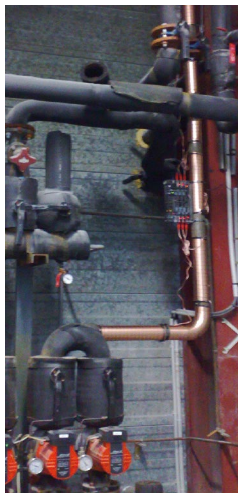
安装在Avignon陶瓷厂的Vulcan S100系统
