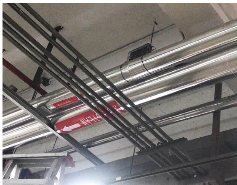
步骤2：管道包裹保温棉，再装上S25主机
