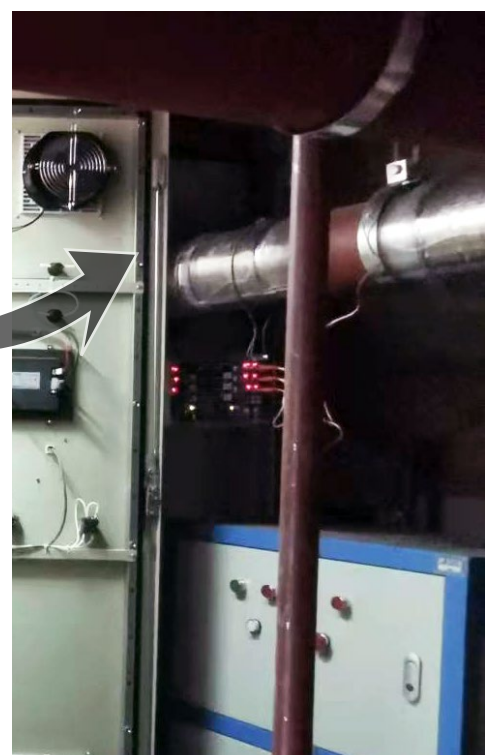
第2步：将Vulcan S100安装在 水管上并包裹脉冲带保护层
