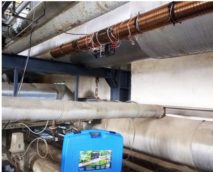
Vulcan S150 安装在主水管上
