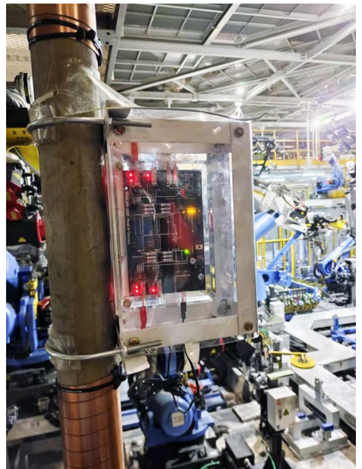
Vulcan S25 安装在机器人循环水系统总管径上
