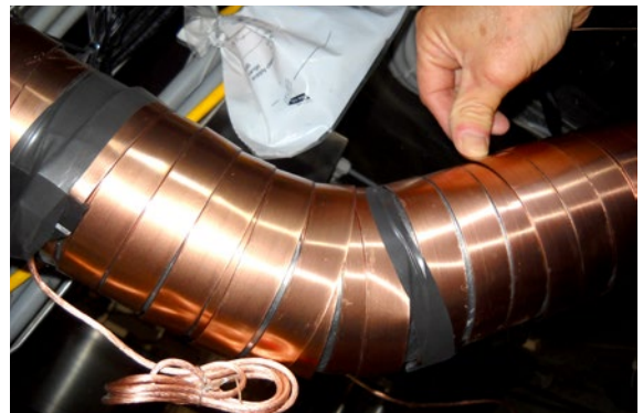
在水管上缠绕了两层的沃肯(Vulcan)脉冲电缆
