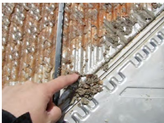
板式换热器上的水垢变软
