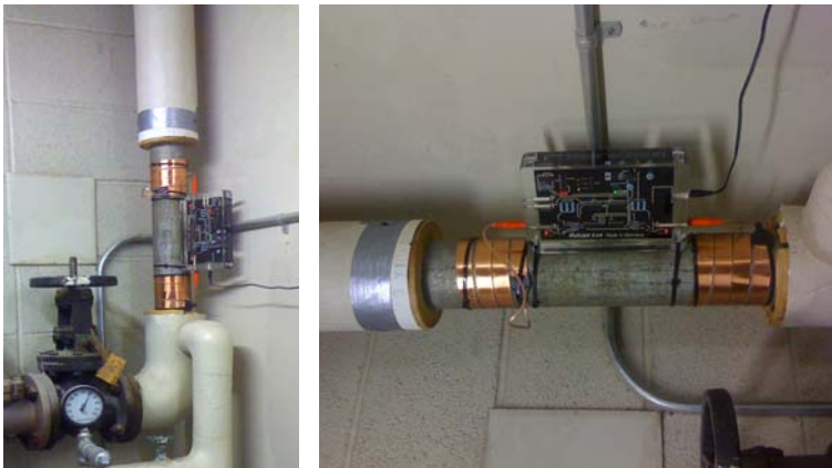
沃肯 (Vulcan) 抑垢除锈装置安装在罗斯福学校整栋建筑主水源
