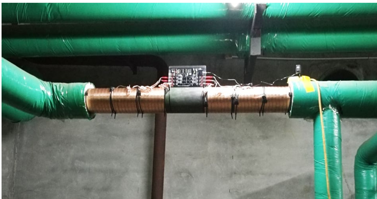
Vulcan S100安装于换热站内低温热水的循环管网主管道上，其补水水源为市政自来水
