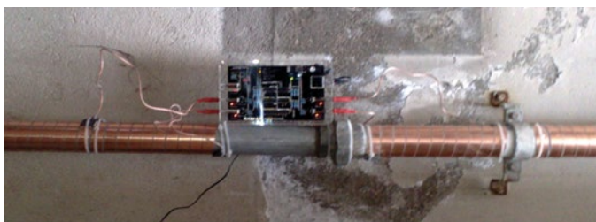
El Vulcan S100 instalado en la fábrica de aluminio Alcoa en Francia
