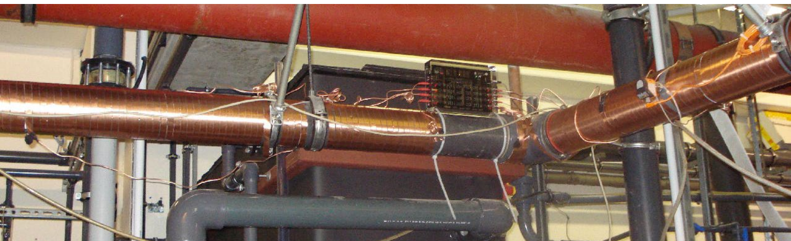
Vulcan S250 tratamiento de tuberías principales de agua para la piscina y la zona de Spa Meridan
