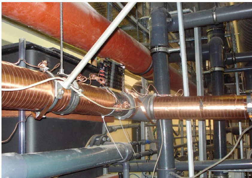
Vulcan S250 tratamiento de tuberías principales de agua para la piscina y la zona de Spa Meridan
