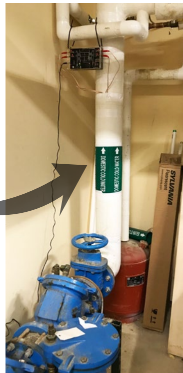
Paso 2: se instaló el equipo S25 en el conducto de agua y se cubrió con la capa protectora
