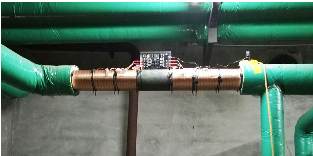
Vulcan S100 se instaló en el suministro principal para la circulación del agua, que proviene del agua municipal.
