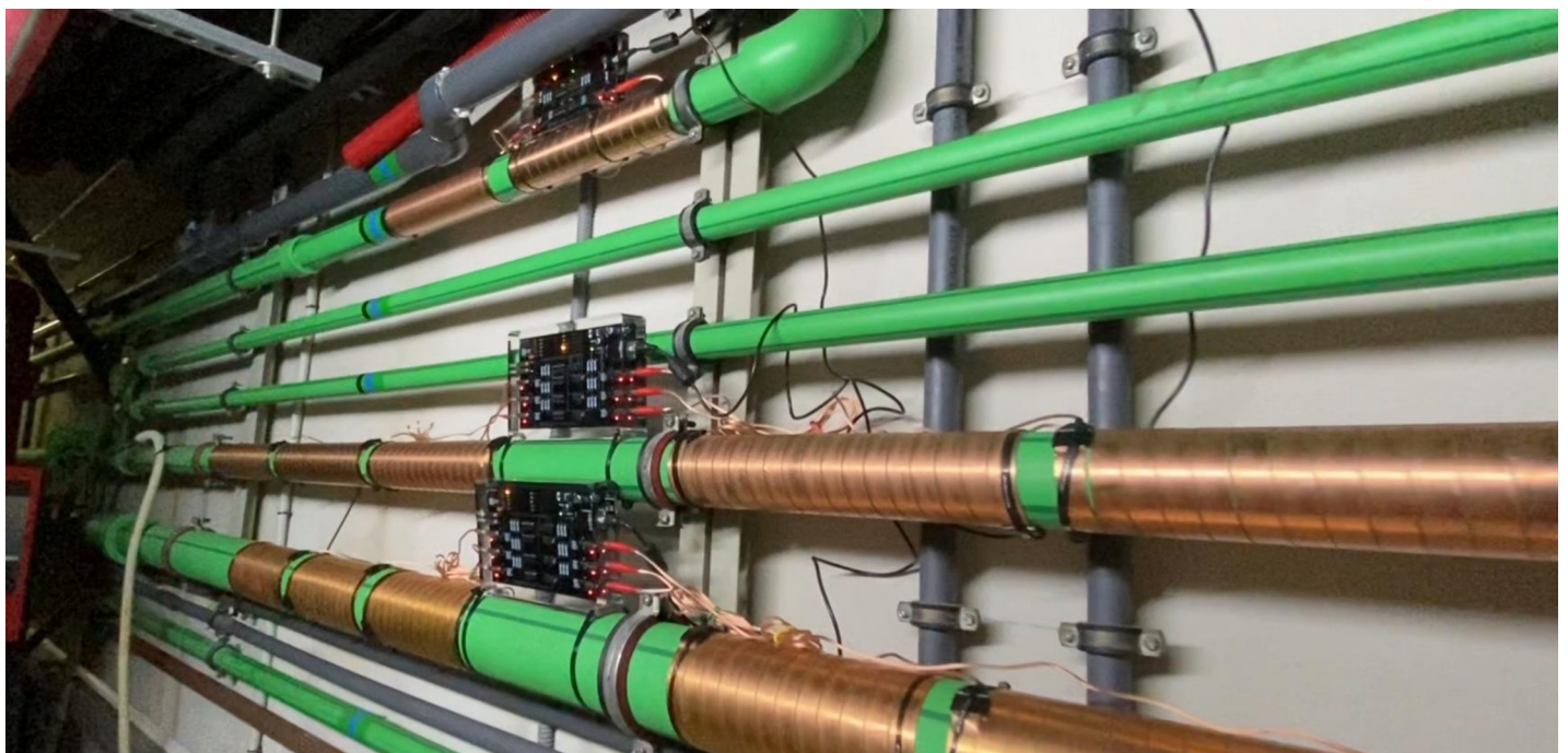
Vulcan S10: En el tubo de agua para el riego con Ø 63 mm
