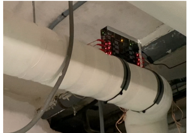
Vulcan S100 En el circuito de agua caliente Ø 110 mm
