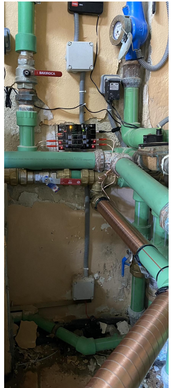
Vulcan S50 en el tubo de agua fría con Ø 63 mm
